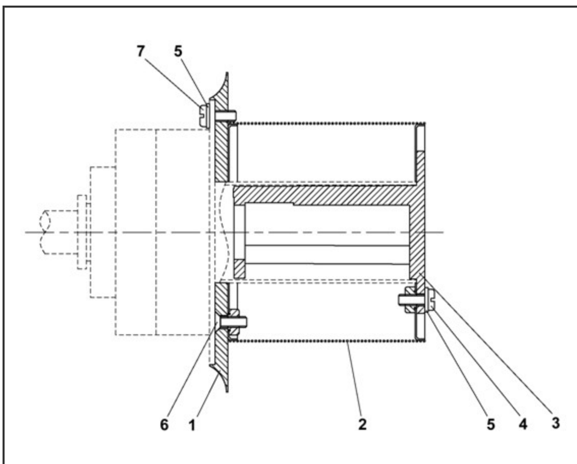
Fig. 8– Kit defletor de ar
