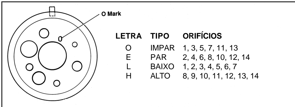
Fig. 7 – Placas alternativas do VRU
