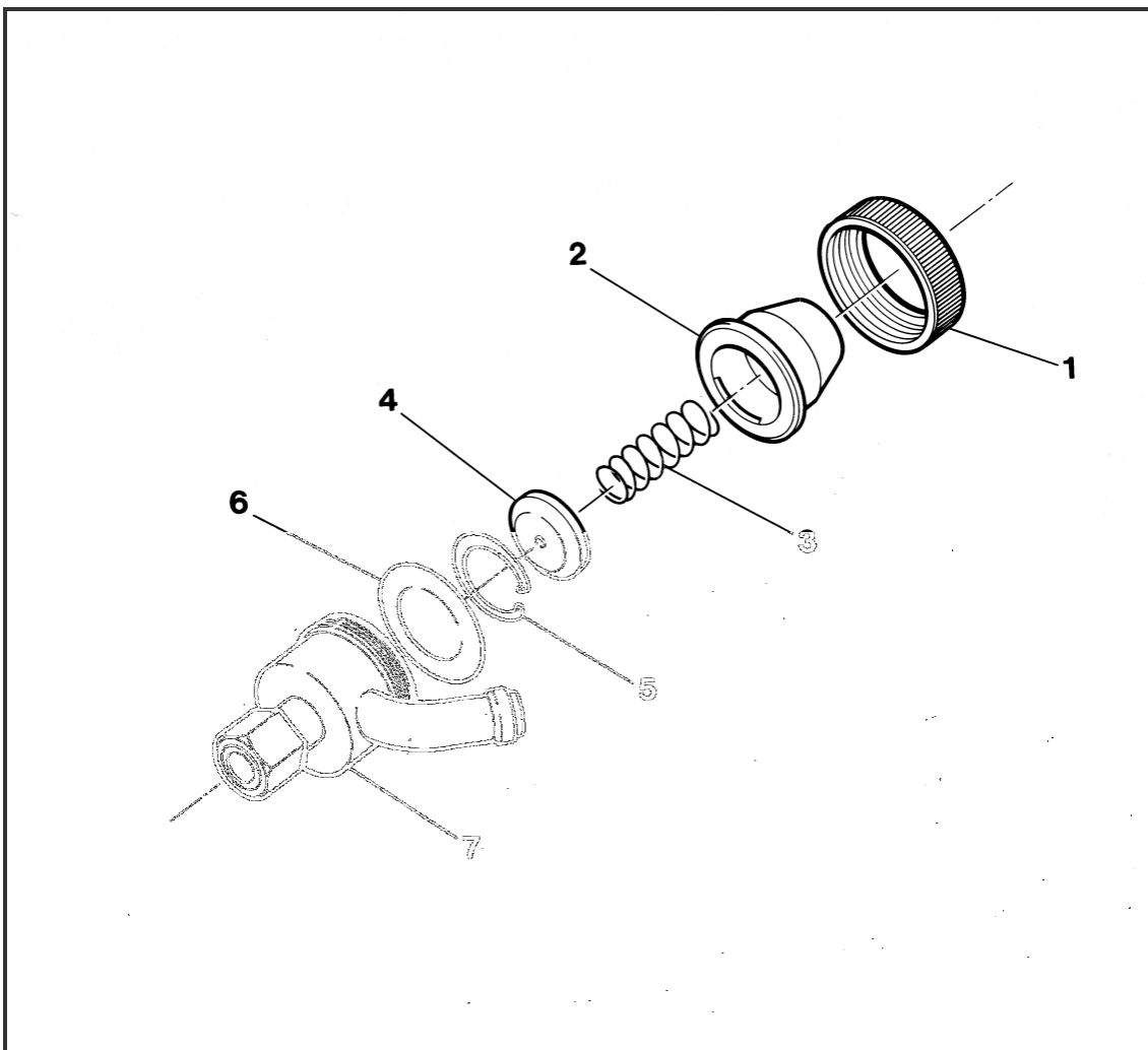
Fig. 11 – Válvula de diafragma
