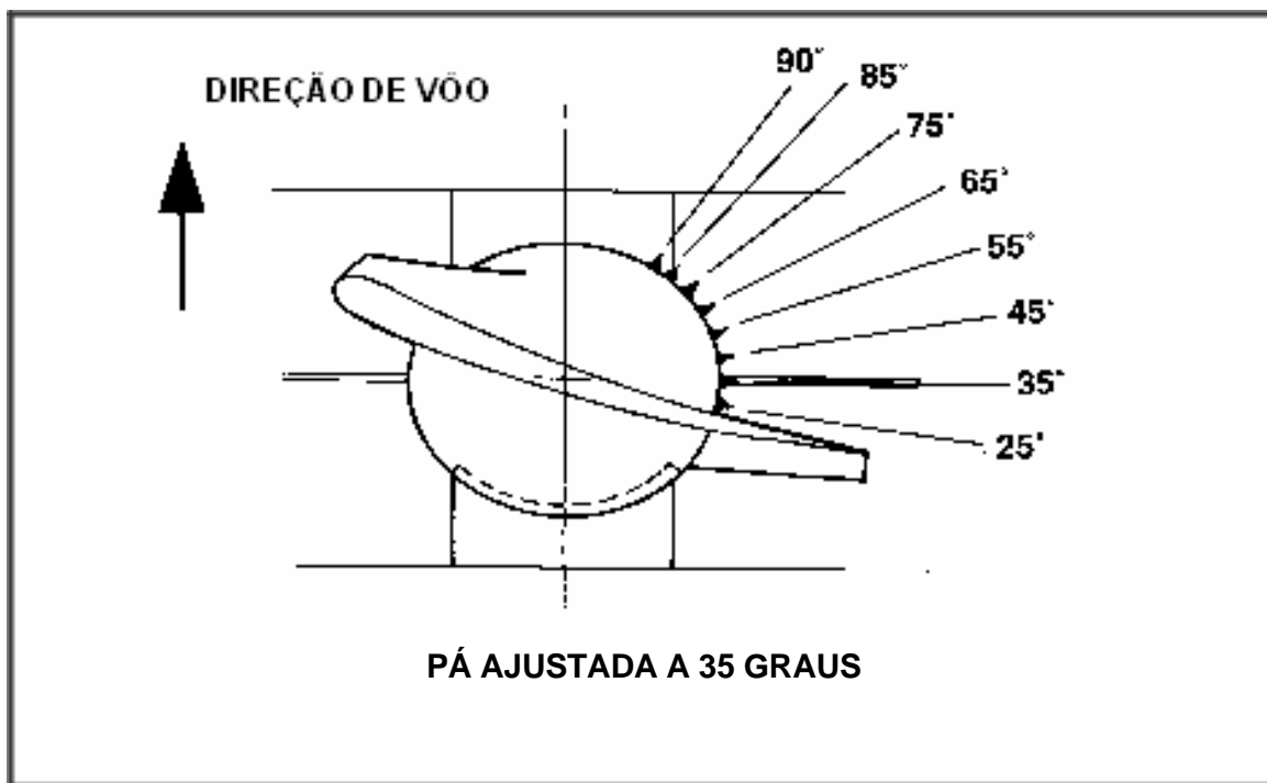
Fig. 5 – Ajuste do ângulo das pás
