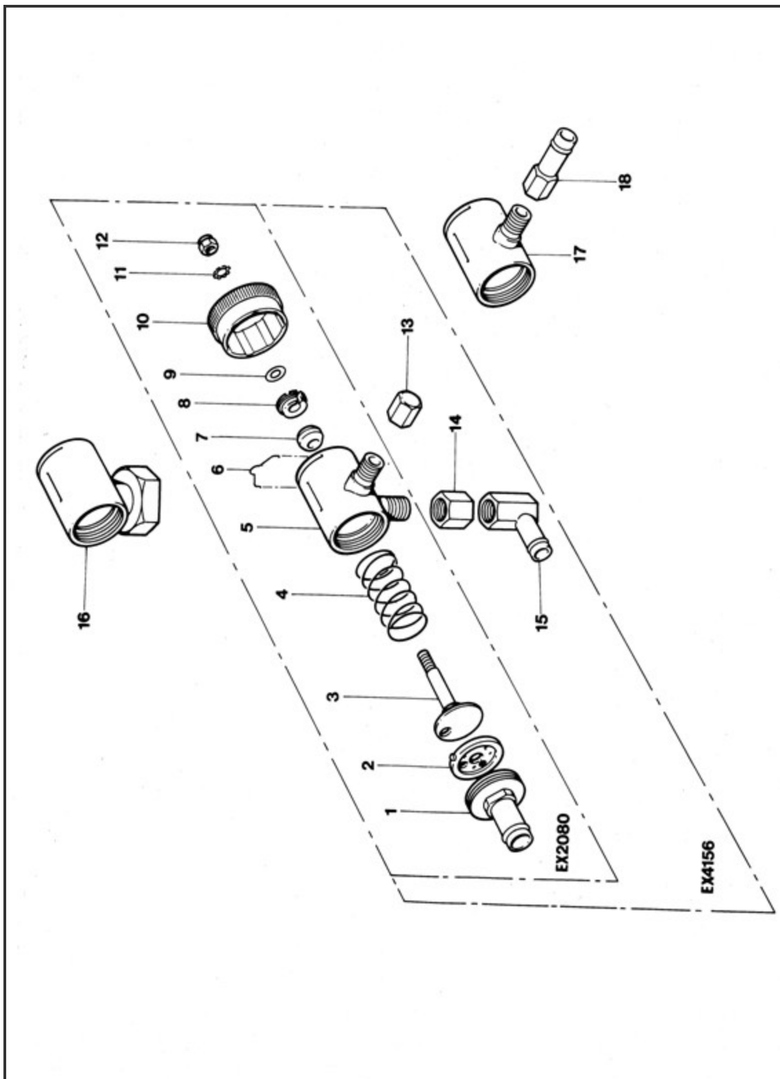
Fig. 10 – Unidade de Restrição Variável e Acessórios Opcionais.
