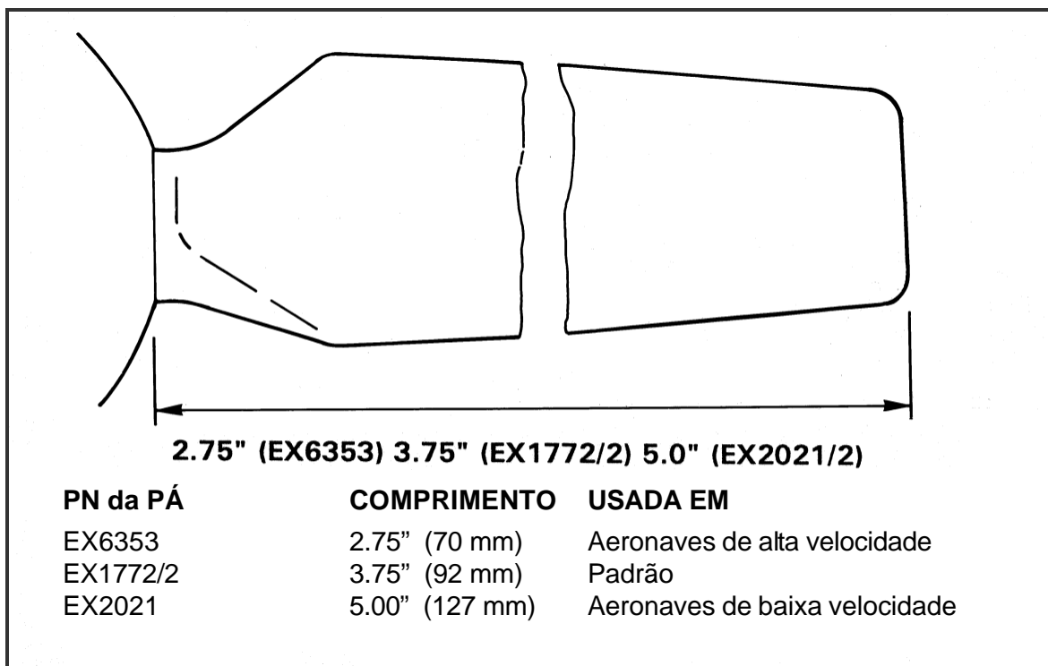
Fig. 6 – Dimensões das pás EX1772/2, EX2021 e EX6353 .
