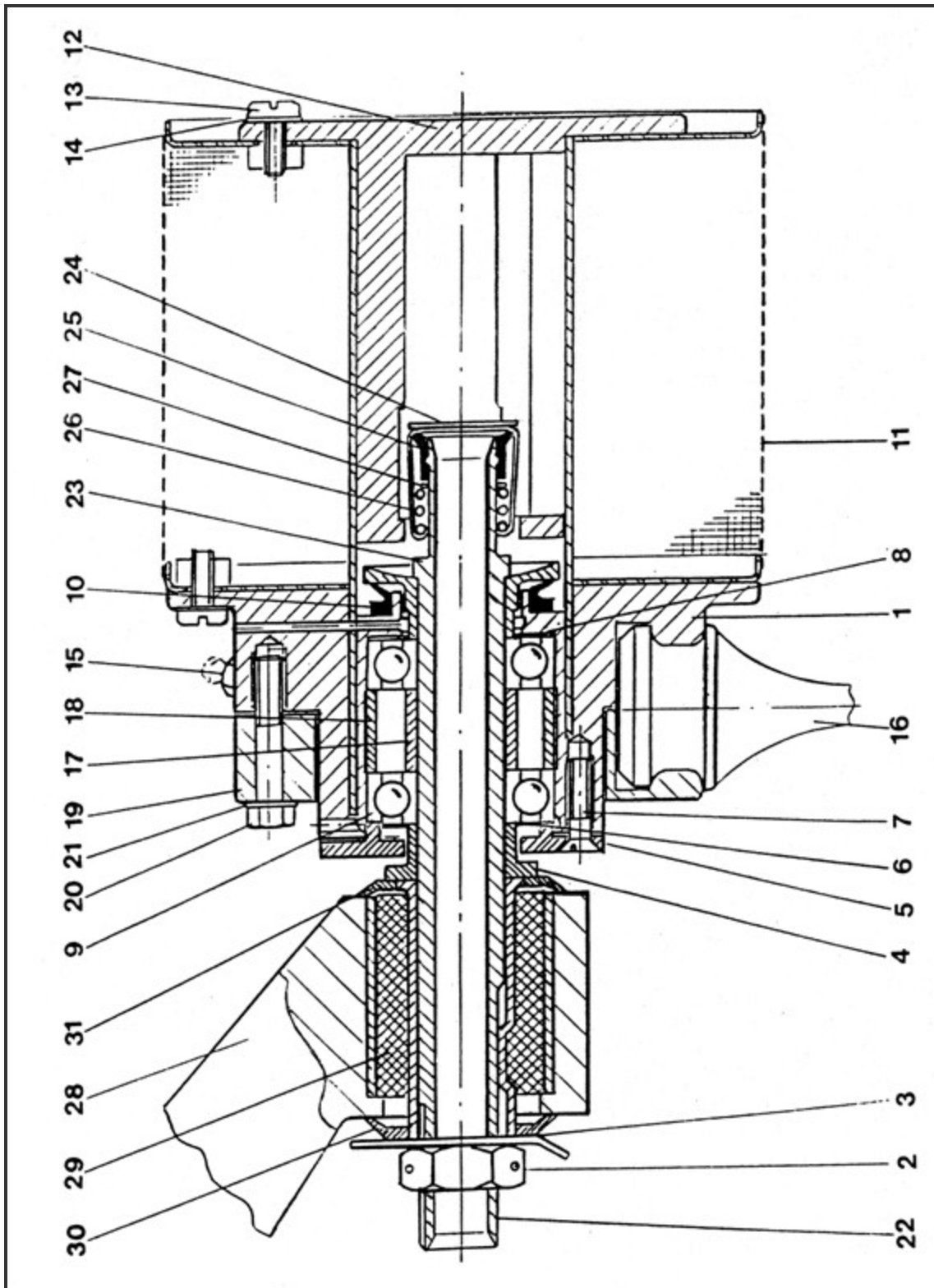
Fig. 9– Atomizador AU5000
