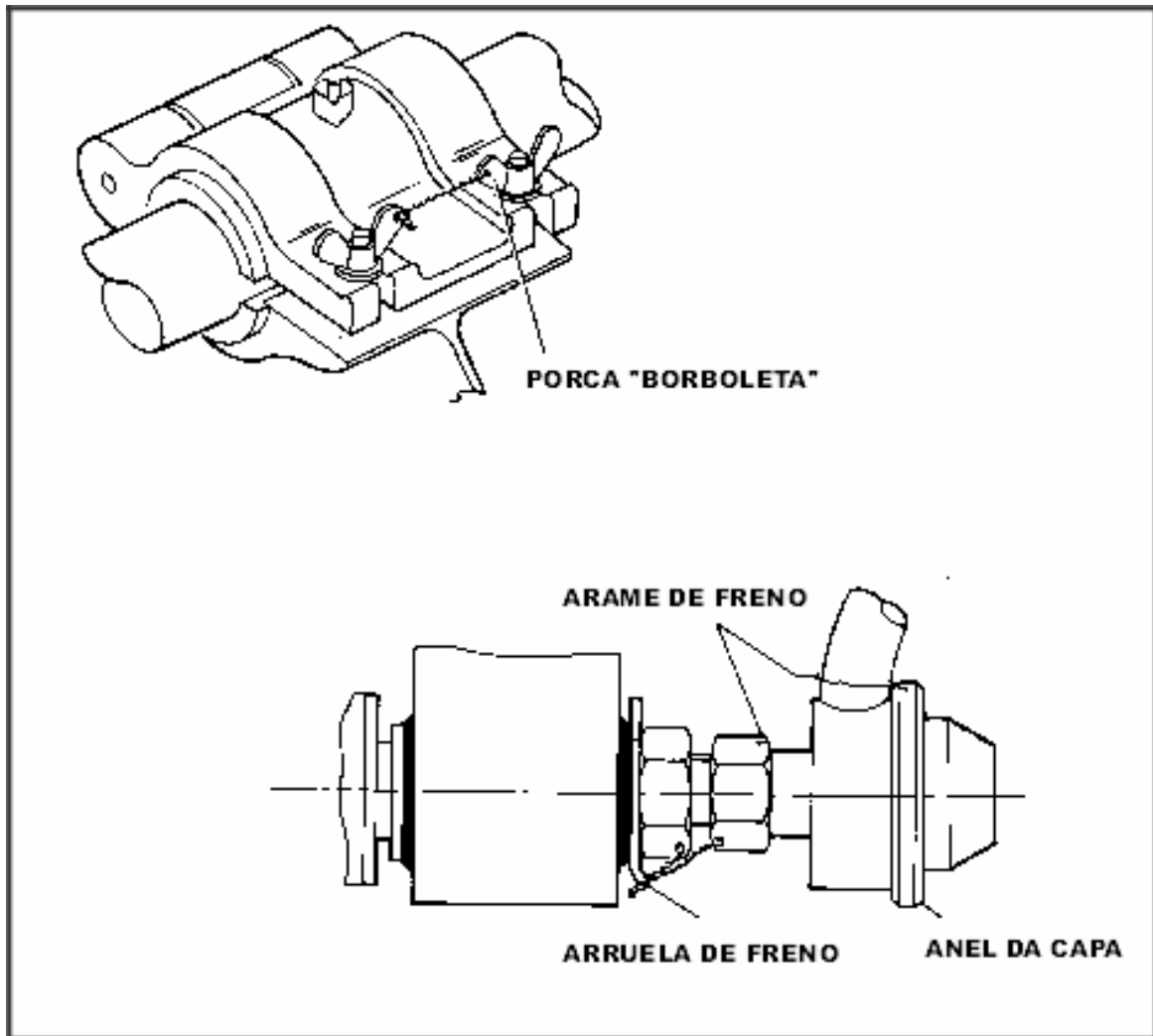
Fig. 2 – Frenagem do atomizador e seus componentes
