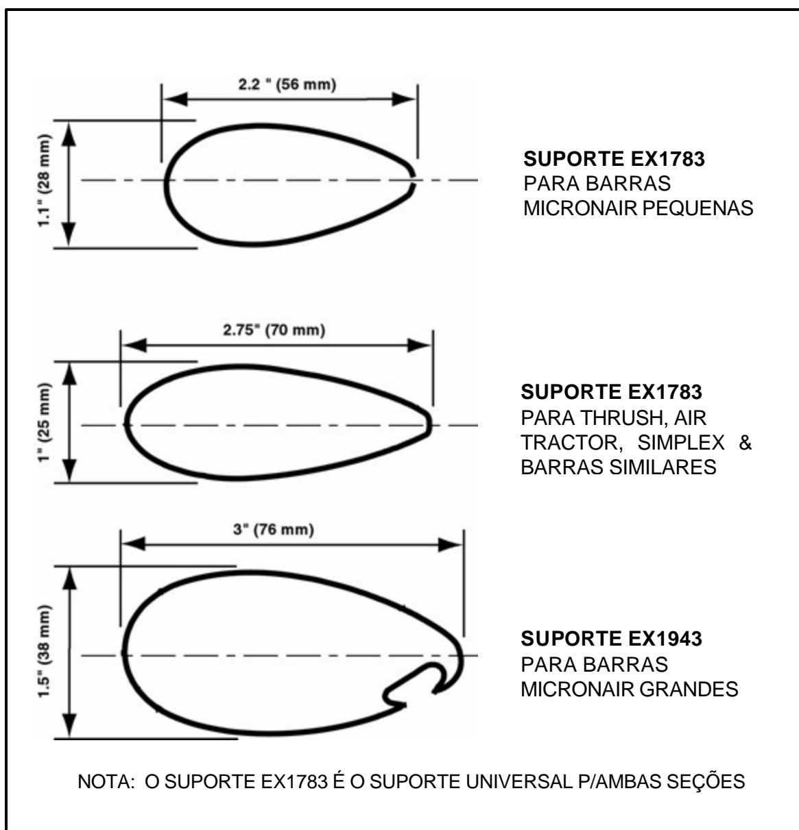
Fig. 3 – Dimensões de suportes para barras aerofólicas
