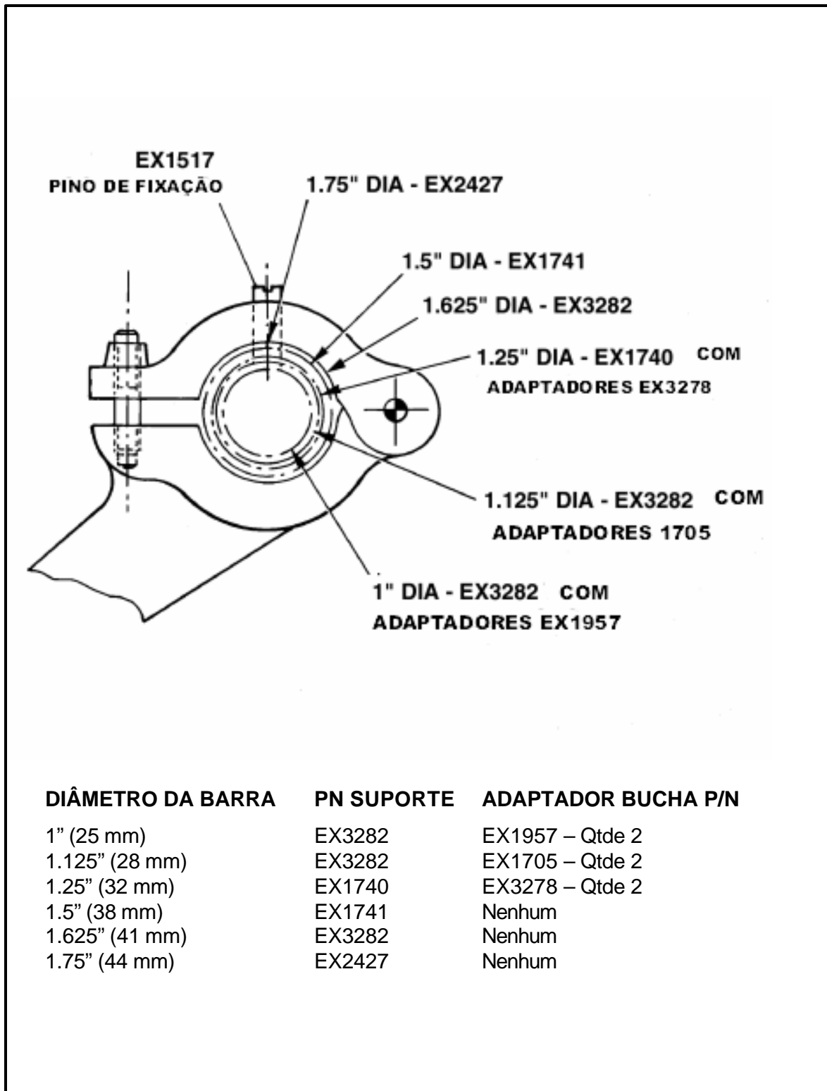
Fig. 4 – Suportes para barras redondas
